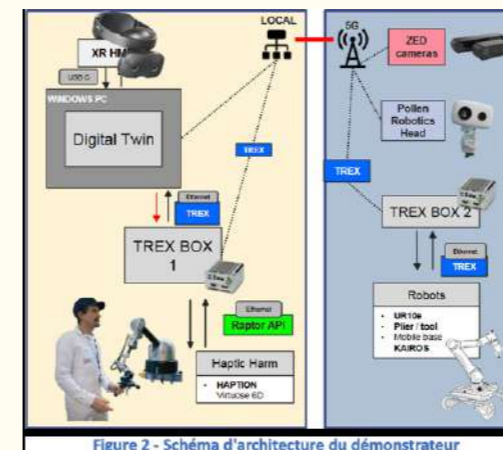
Figure 2 - Schéma d'architecture du démonstrateur
