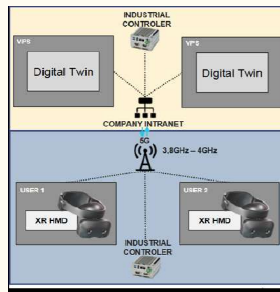
Figure 1 - Schéma d'architecture du usecase Simulation Immersive
