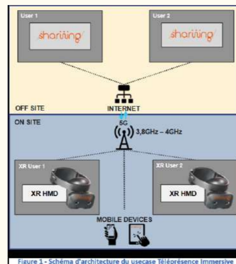
Figure 1 - Schéma d'architecture du usecase Téléprésence Immersive
